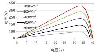
P-V曲线
