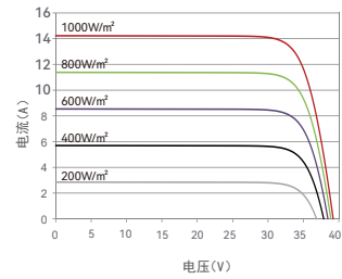
I-V曲线
